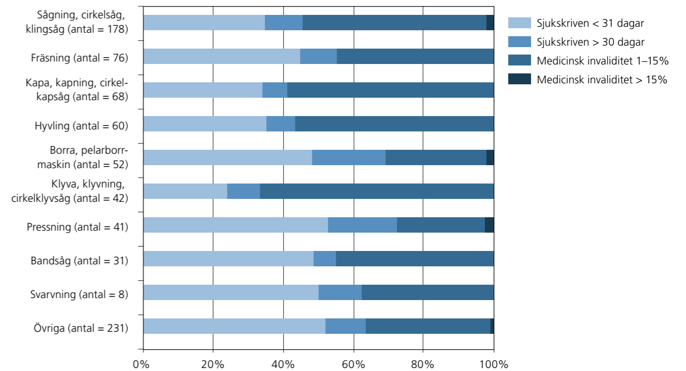
Diagram 19. Maskinolycksfall i trämanufakturverksamhet. Fördelning på typ av bearbetning/maskin och skadans allvarlighet. Antal = 786.
